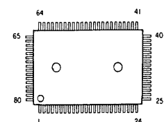
CXD2526Q
