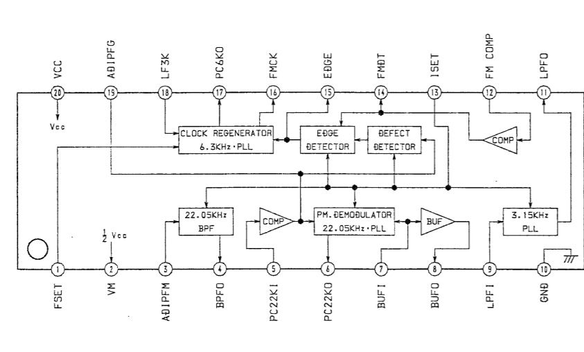
IC161 CXA1380N
