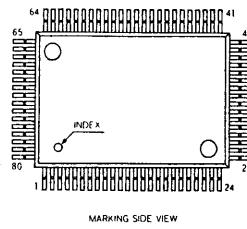
M38067M8-051FP
