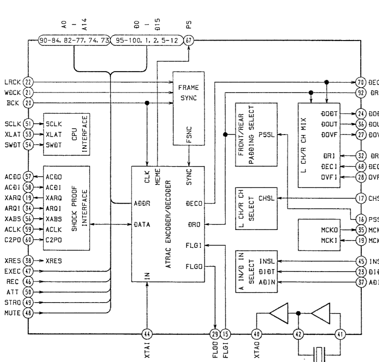
IC102 CXD2527R-1
