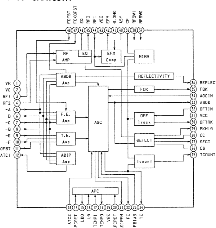
IC209 CXA1381R
