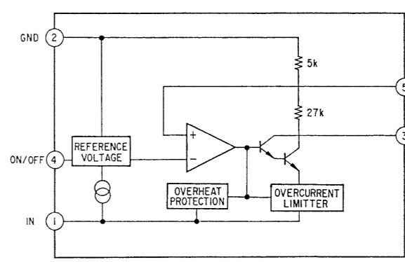
IC501 M5293L
